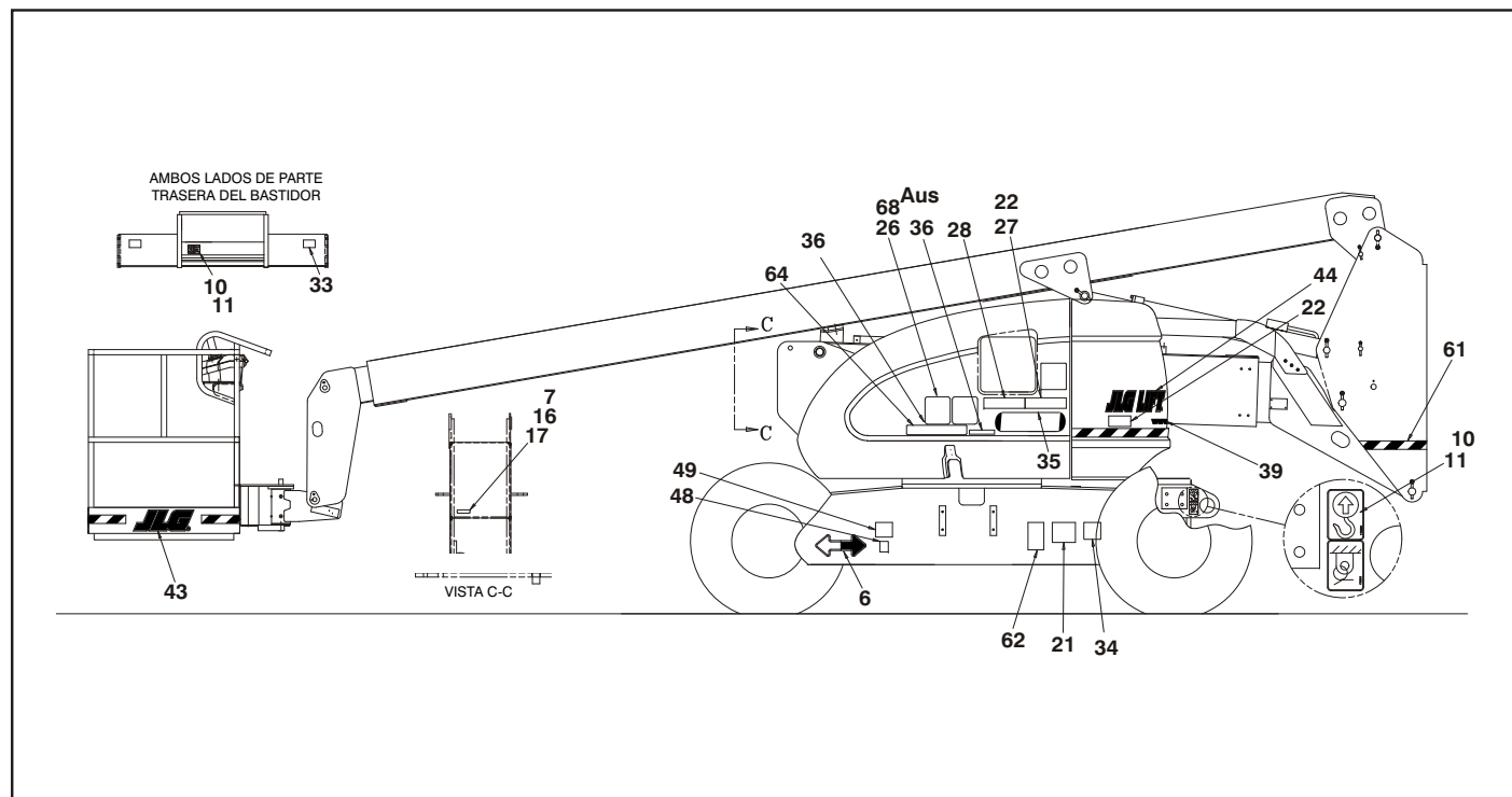
Figura 4-10. Instalación de etiquetas en 600A y 600AJ
