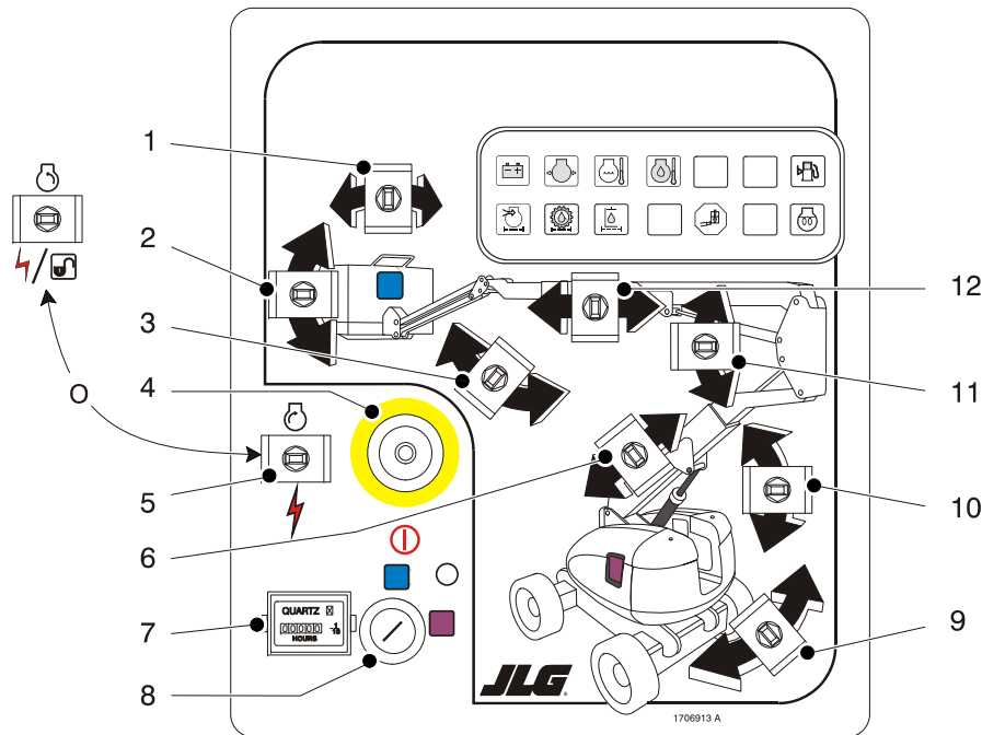
Figura 3-1. Puesto de controles de suelo
