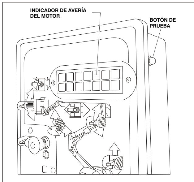
Figura 3-3. Indicador de avería y botón de prueba
