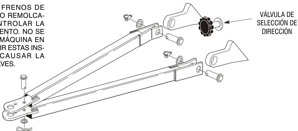
Figura 4-5. Puntos de conexión de barra de remolcado - Máquinas con NS anterior al 81836
